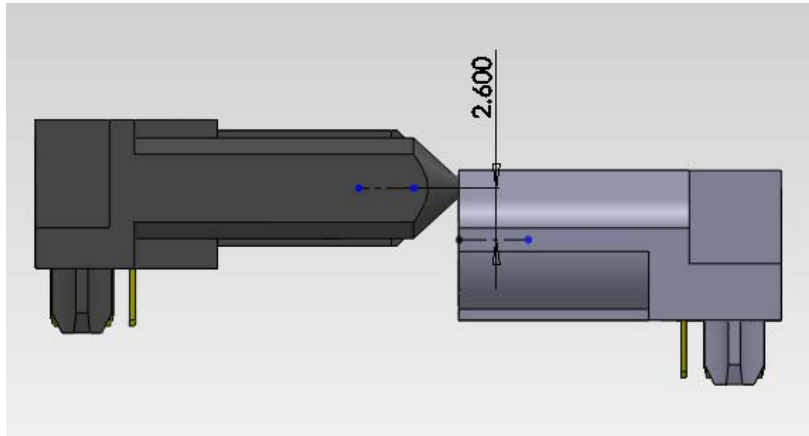
allowed misalignment in transverse axes 在橫向方向允許對插偏差量
