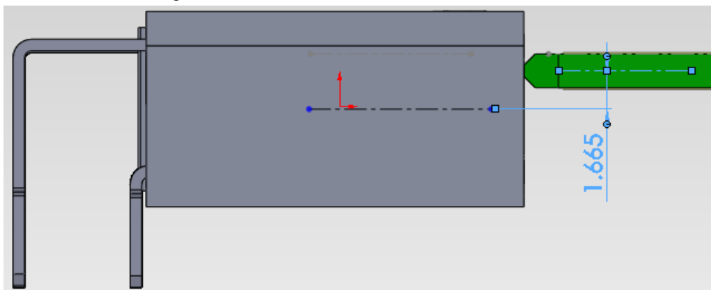
allowed misalignment in longitudinal axes 在縱向方向允許對插偏差量
