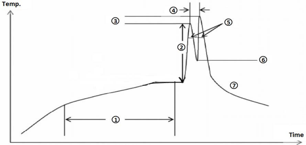
附表三：波峰焊曲線圖
