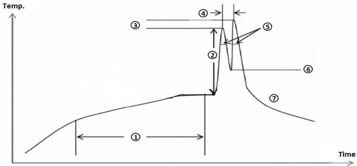
附表三：波峰焊曲線圖
