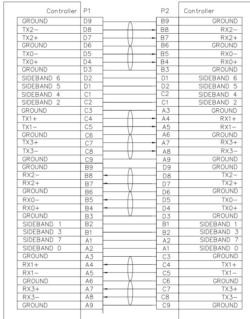
WIRING TABLE
