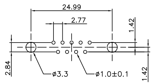
P.C.Board Layout
