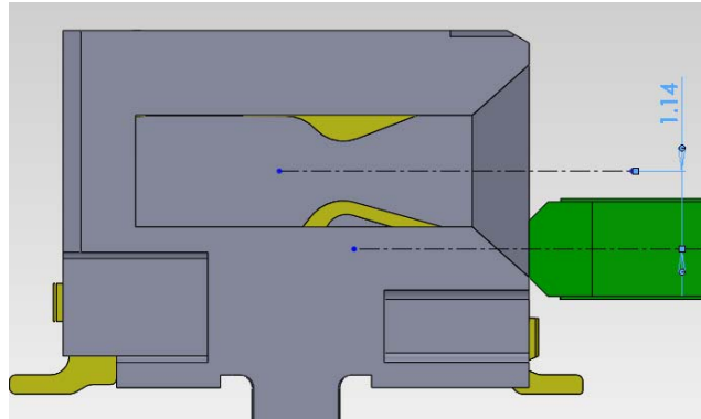
allowed misalignment in transverse axes 在橫向方向允許對插偏差量
