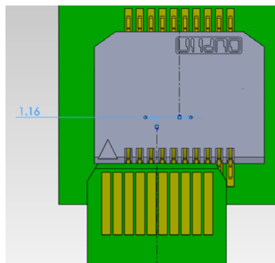
allowed misalignment in transverse axes 在橫向方向允許對插偏差量
