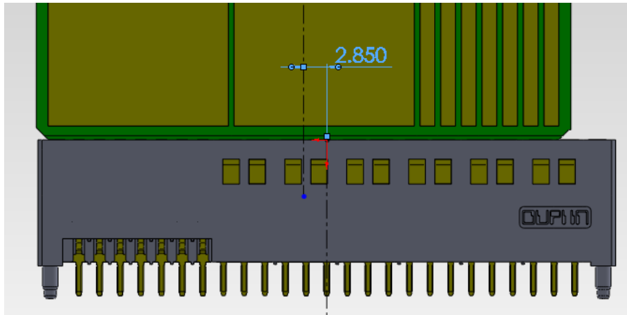
allowed misalignment in transverse axes 在橫向方向允許對插偏差量
