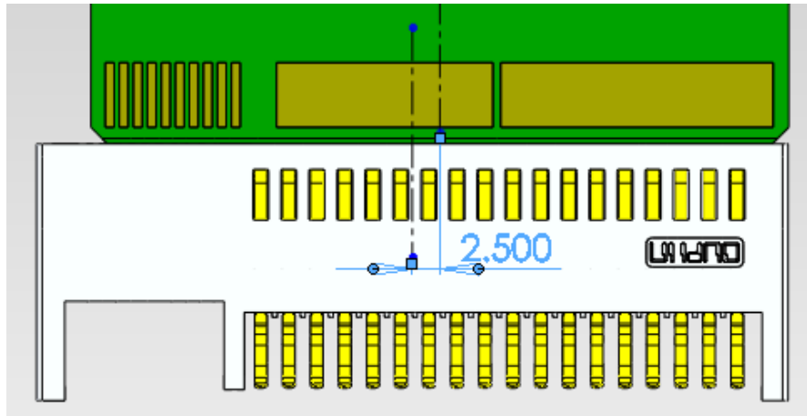
allowed misalignment in transverse axes 在橫向方向允許對插偏差量
