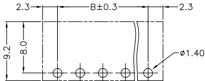
P.C.Board Layout
