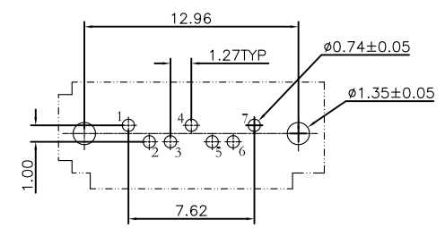
P.C.Board Layout
